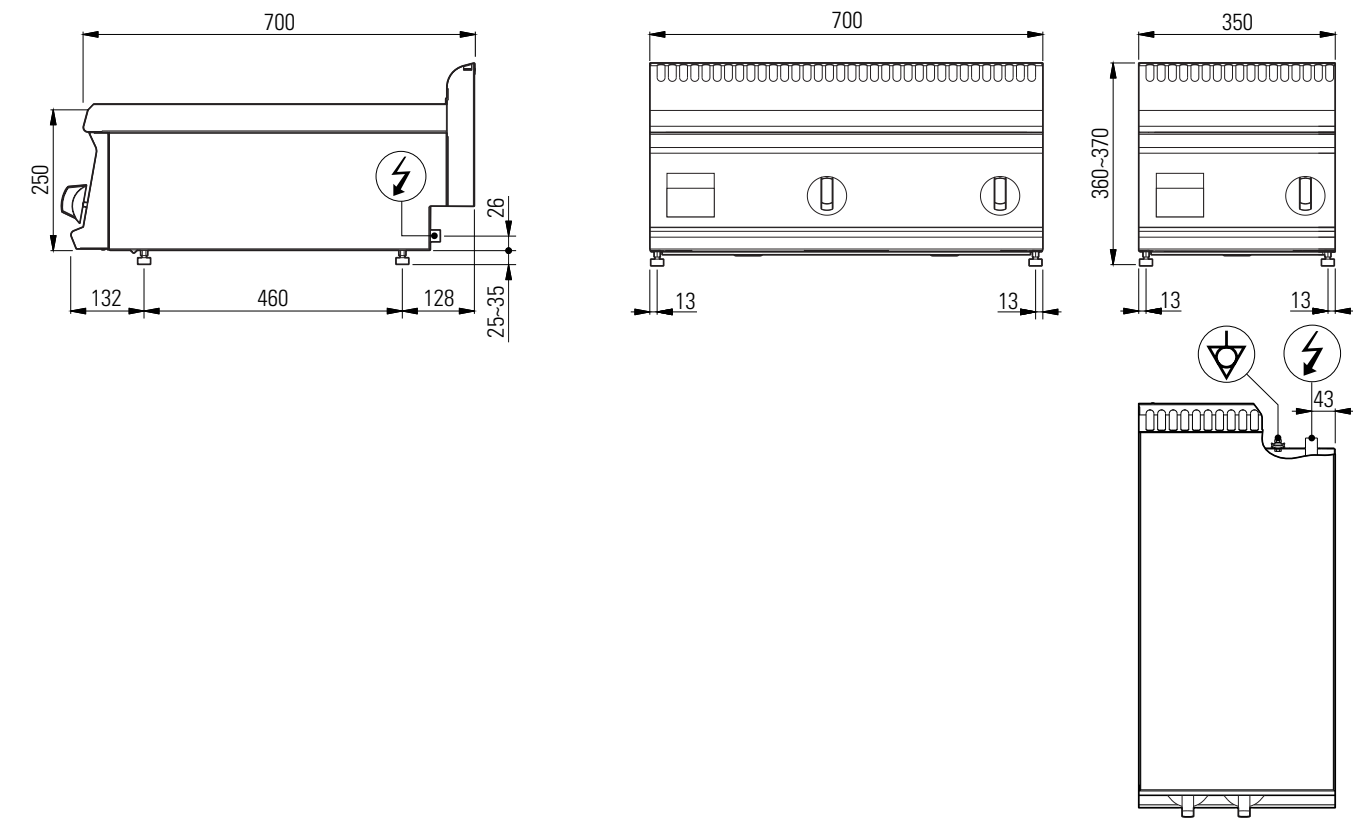
Fig.1 | Abb.1 | рис.1 - 5416.162.00
