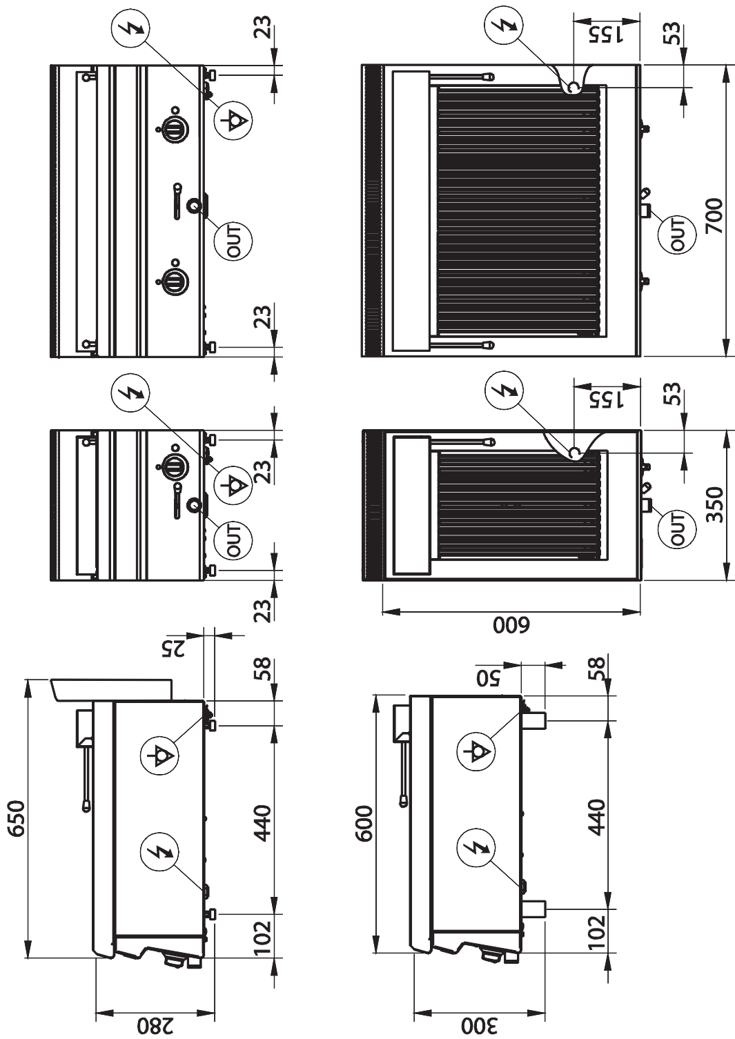
Fig.1 | Abb.1 | рис.1 - 5415.687.00
