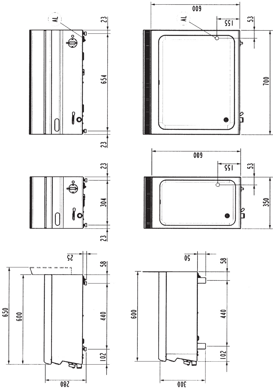
Al = Entrada cavo elettrico | Power supply cable inlet | Netzkabeleingang | Вход электропровода | Entrée cable électrique | Entrada cable eléctrico.
