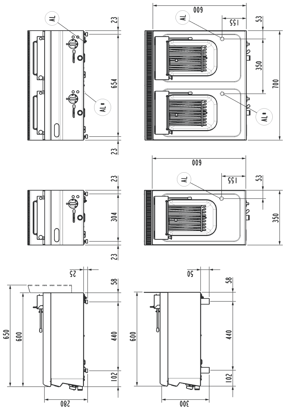
AL = Entrata cavo elettrico | Power supply cable inlet | Netzkabeleingang | Вход электропровода | Entrée câble électrique | Entrada cable de alimentación. AL* = Entrata 2° cavo elettrico | 2nd Power supply cable inlet | 2° Netzkabeleingang | 2° Вход электропровода | Entrée 2° câble électrique | Entrada 2° cable de alimentación.
