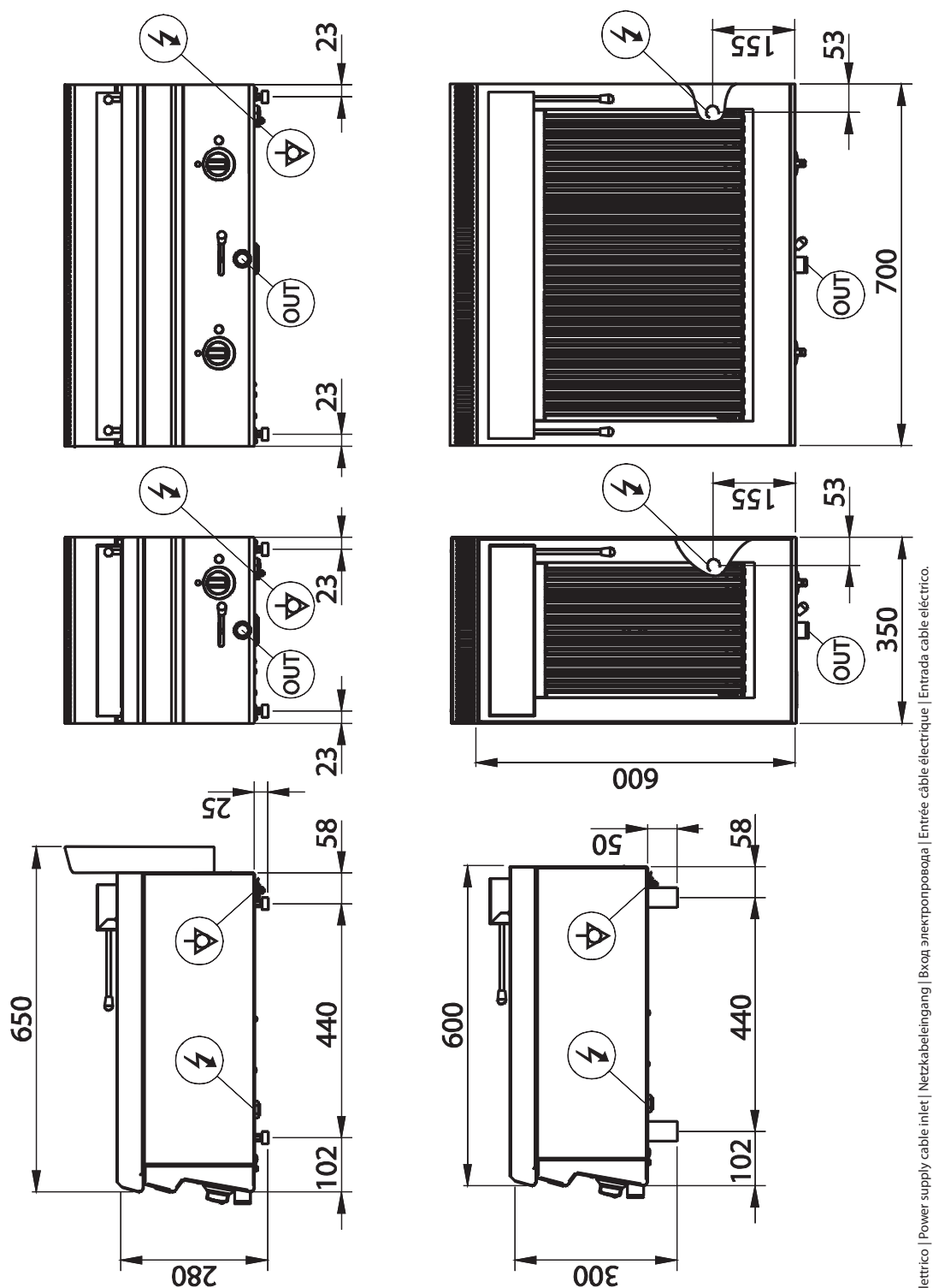
Fig.1 | Abb.1 | рис.1 - 5415.687.00
